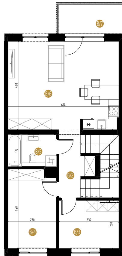
1 PIĘTRO
